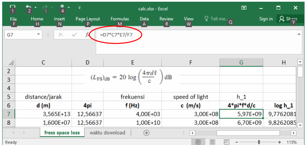
Gambar-1 . calculated cell pada excel
